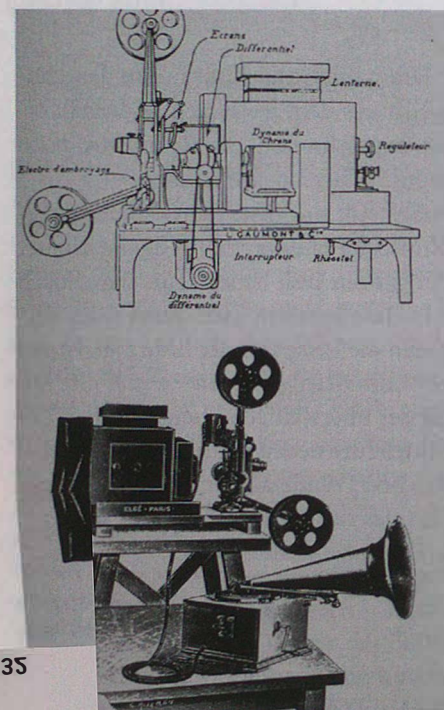
1. Chrono-5 (H 2 -Projektionssystem „Chrono-5“ von der Firma Gaumont, Paris 1902)
